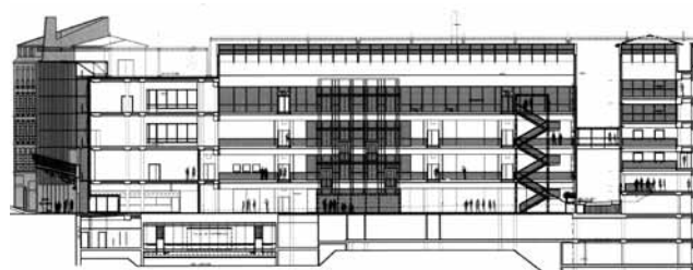
COUPE LONGITUDINALE
